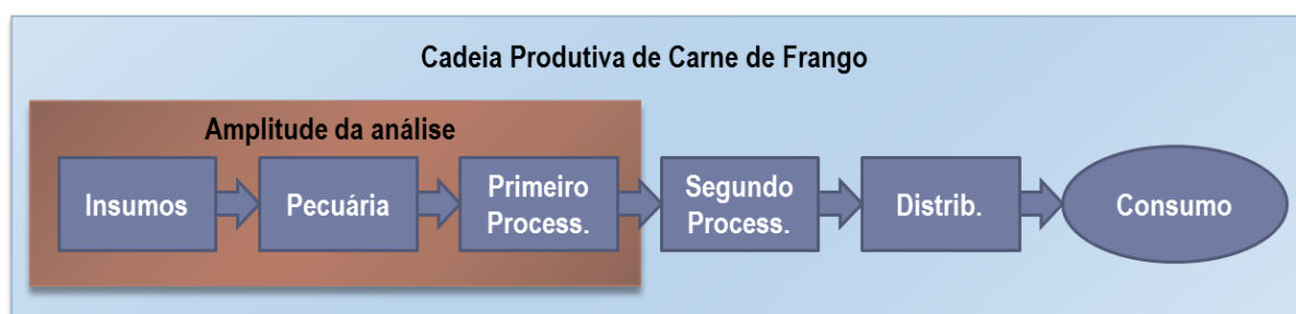
Figura 1 – Amplitude da análise de transmissão de preços
