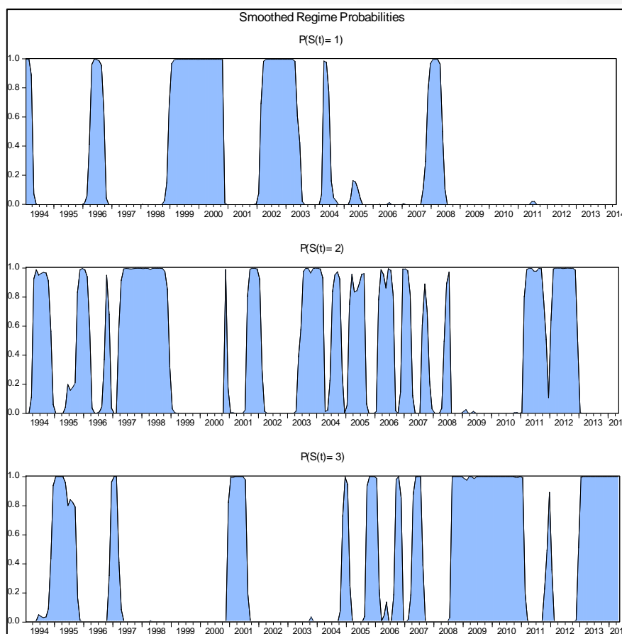
Figura 3 – Períodos de permanência em cada regime
